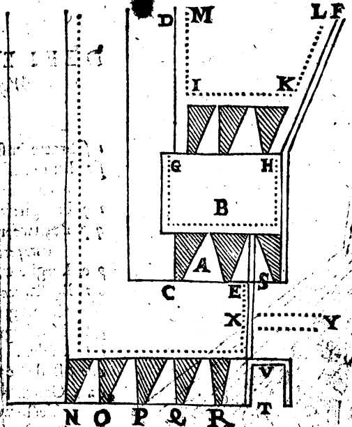
DEELEN DER 3 e FORM, Wesende grontteyckening van een stryck- bouck met haer drie plaetsen.
