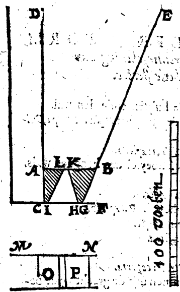
DEELEN DER 2 e FORM, Wesende grontteyckening van een stryckbouck met haer middelplaets.
